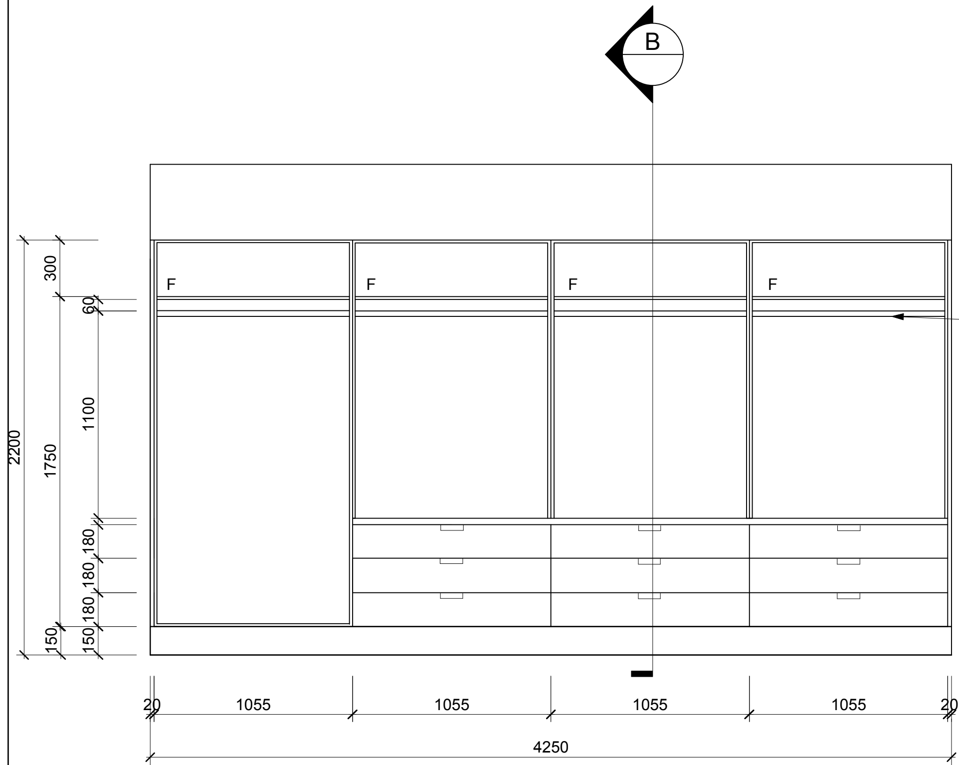
ELEVATION
